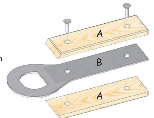
Explosie - overzicht
